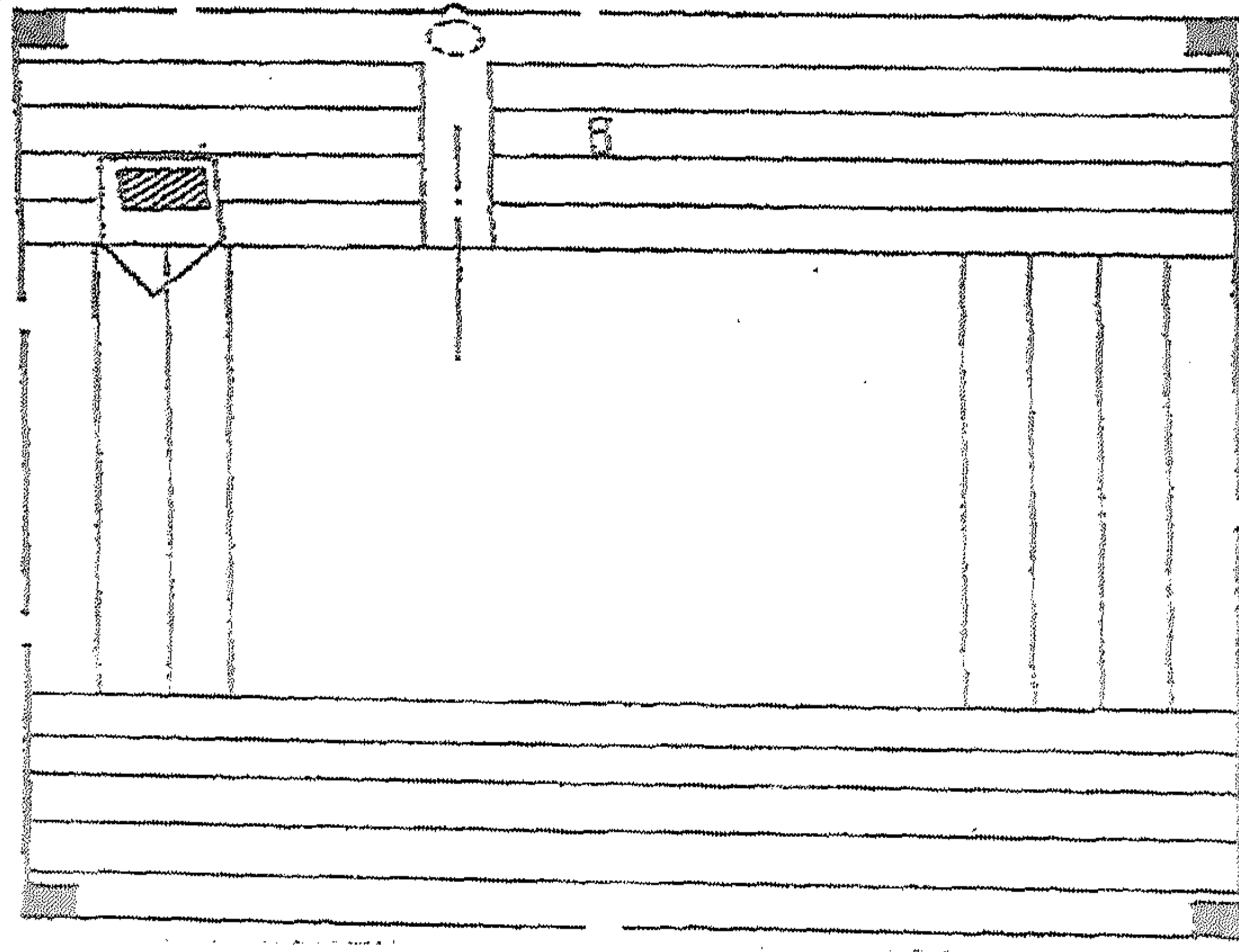
(شكل رقم ٨٩) رسم تخطيطي لمسجد الرسول صلى الله عليه وسلم بالمدينة في عهد الوليد بن عبد الملك عن أيزين
